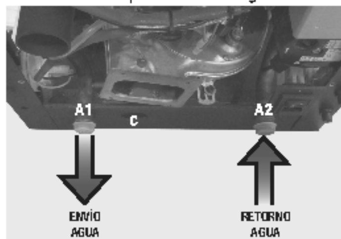
Esquema conexión termo estufa sin kit de producción de agua sanitaria
