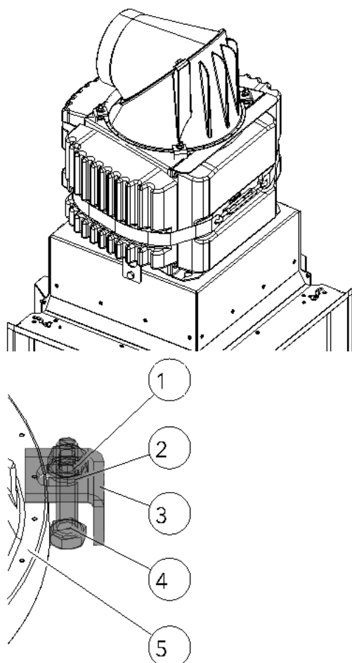
Abb. 39: Abgassammler montieren
