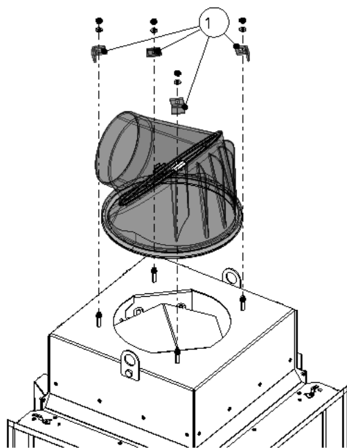
Abb. 40: Rauchsammler abmontieren
