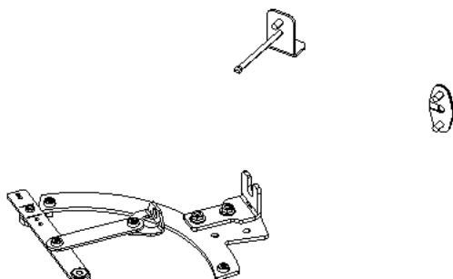
Abb. 53: Montageset 363005
