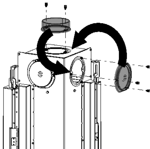
Abb. 32: Teile tauschen
