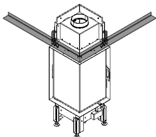
Abb. 75: Tragrahmen montieren
