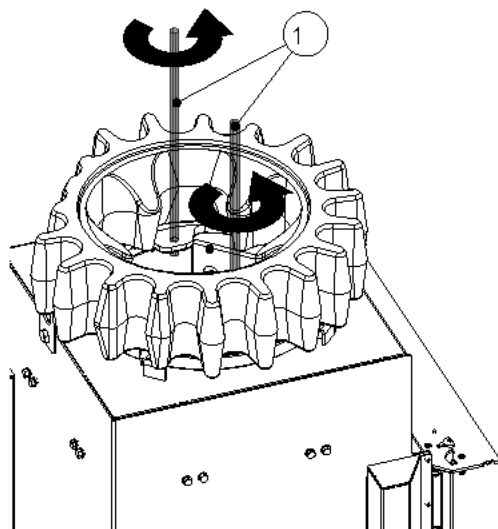
Abb. 47: Gewindestange montieren
