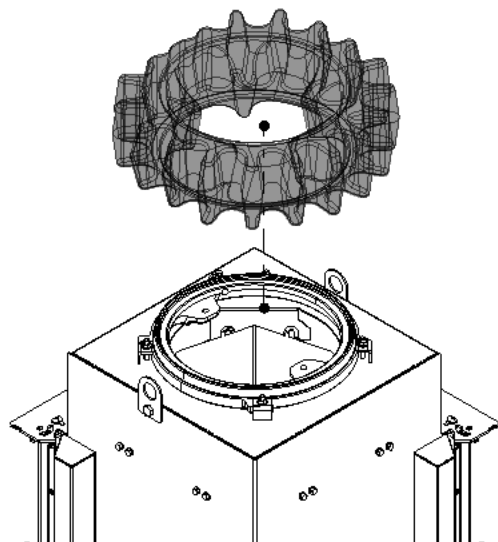
Abb. 46: Aufsatzspeicherstein aufsetzen
