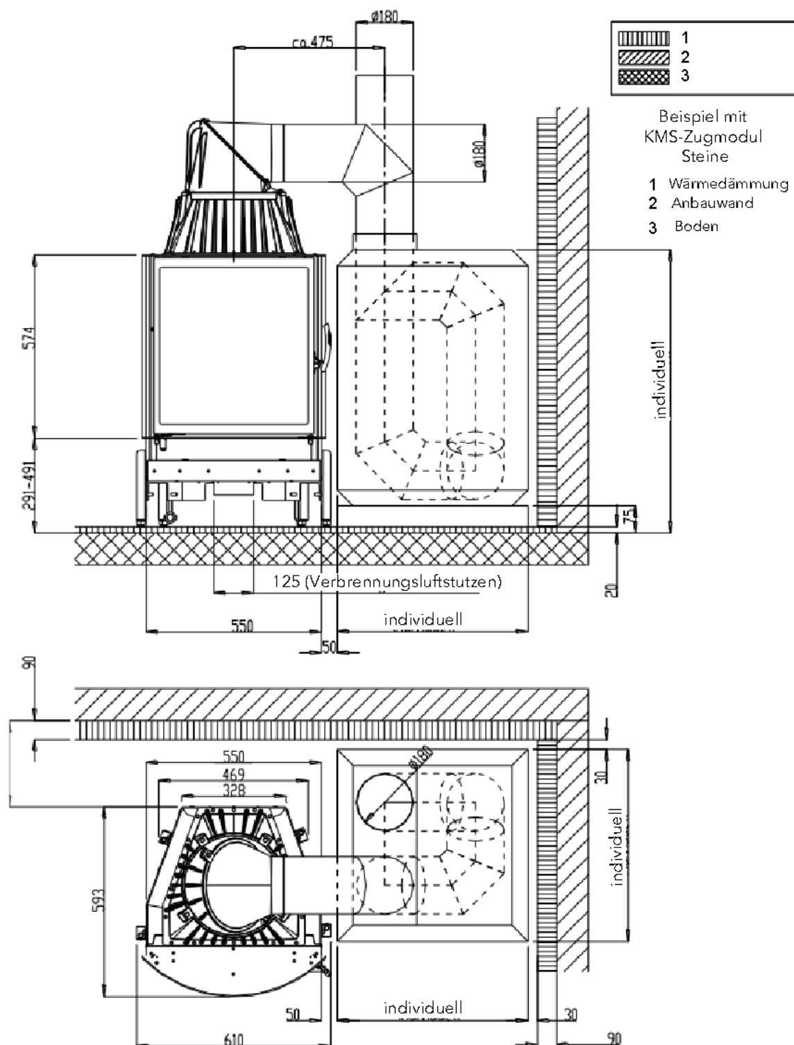
Abb. 15: KMS-System
