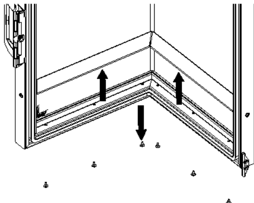
Abb. 29: Reflektoren umbauen
