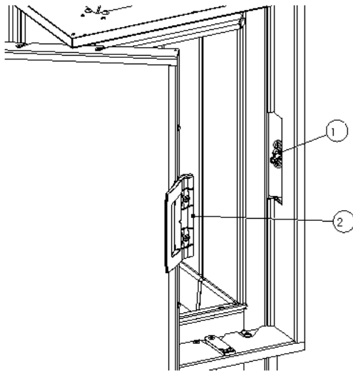
Abb. 79: Tür einstellen
