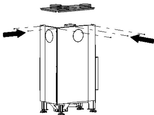
Abb. 71: Deckel vom KV-Mantel befestigen
