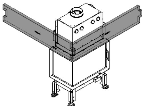
Abb. 76: Tragrahmen montieren
