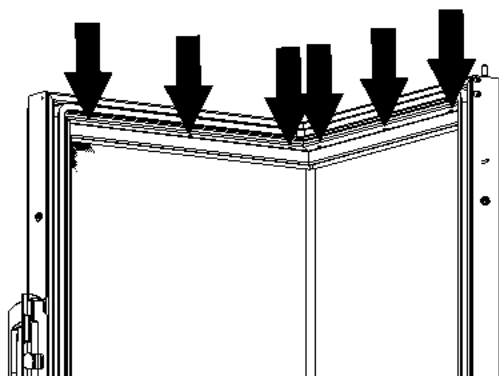
Abb. 28: Gewindestifte rausdrehen
