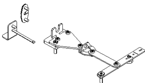
Abb. 50: Steuerungseinheit
