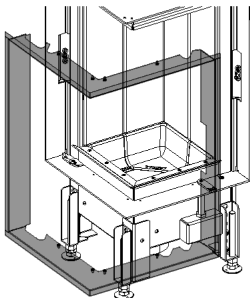
Abb. 74: Designrahmen anbringen und befestigen
