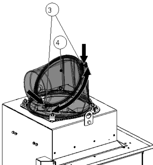
Abb. 81: Rauchsammlerstutzen einstellen
