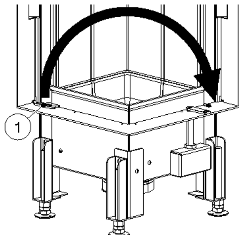
Abb. 26: Abdeckungen ummontieren
