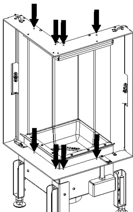
Abb. 73: Schrauben rausdrehen
