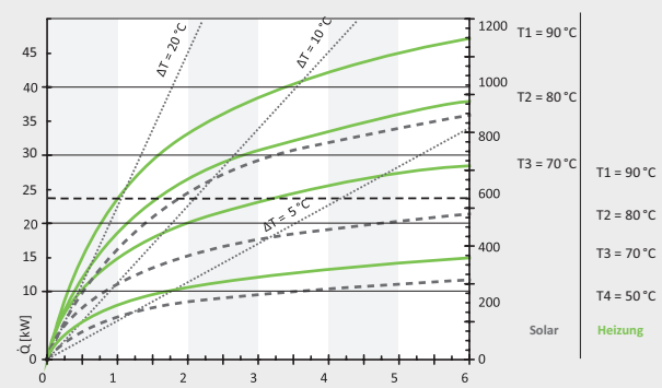
Storatherm Aqua Solar 200/2 bei einer Zapftemperatur von 45 °C
