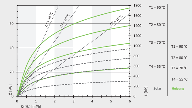
Storatherm Aqua Solar 300/2 bei einer Zapftemperatur von 45 °C
