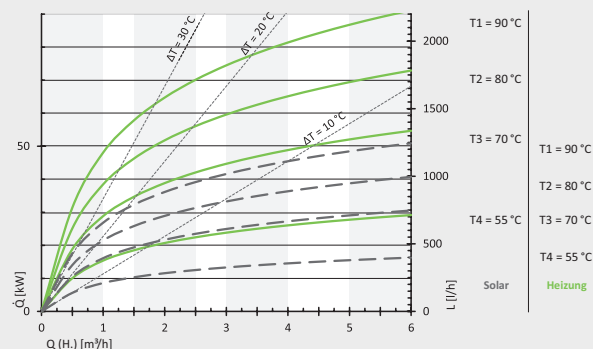
Storatherm Aqua Solar 750/2 bei einer Zapftemperatur von 45 °C
