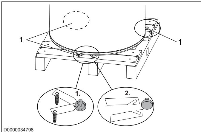
1 Metalllasche mit Schraube
