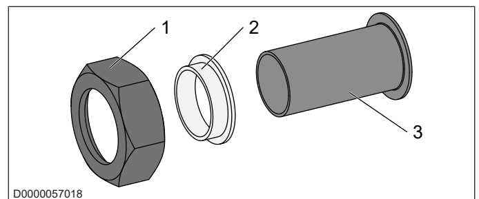
1 Überwurfmutter (G1) 2 Isolierhülse 3 gebördeltes Rohr (22x1 mm, Kupfer)
