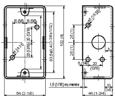
Caixa de distribuição
