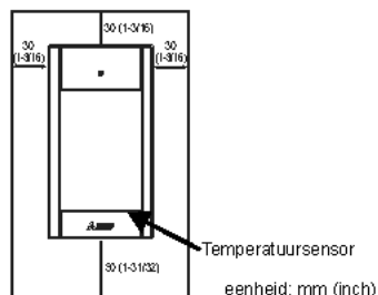
Buitenafmetingen van de afstandsbediening
