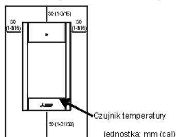
Zewnętrzne wymiary sterownika zdalnego
