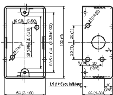
Boîtier de connexion
