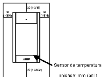
Dimensões externas do controlador remoto
