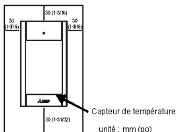
Dimensions externes de la télécommande
