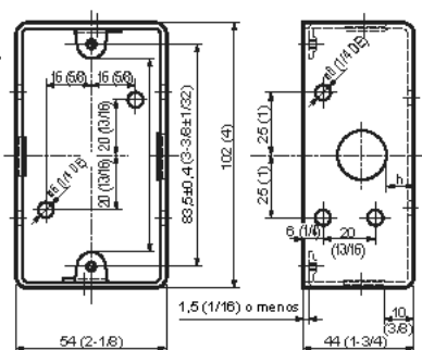
Caja de interruptores
